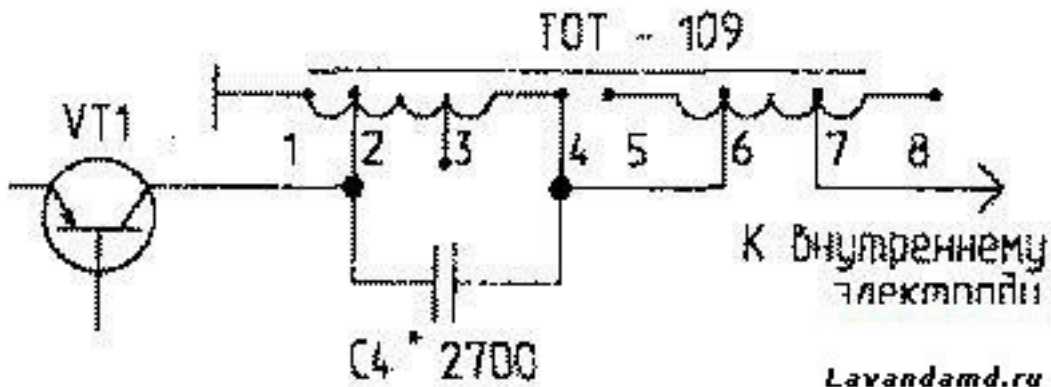
Рис. 5. Вспомогательная обмотка (105 мА) под трансформатор Т0Т-109 приведена на рис. 6.
