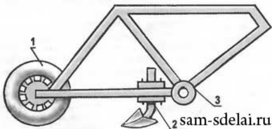
Культиватор (план) для изготовления культиватора (с
